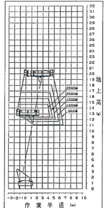
アウトリガ最小張出
