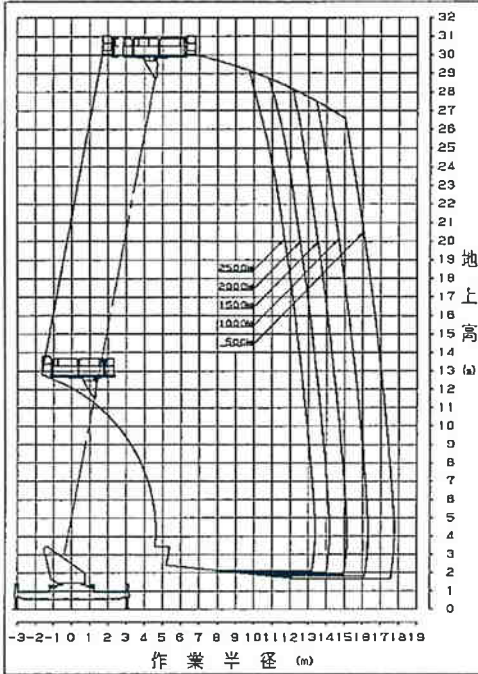
アウトリガ最大張出
