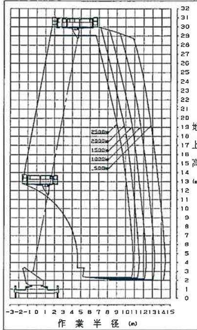
アウトリガ中間2張出
